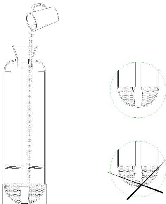
Рисунок 6 — Порядок загрузки фильтрующего материала в корпус фильтра
