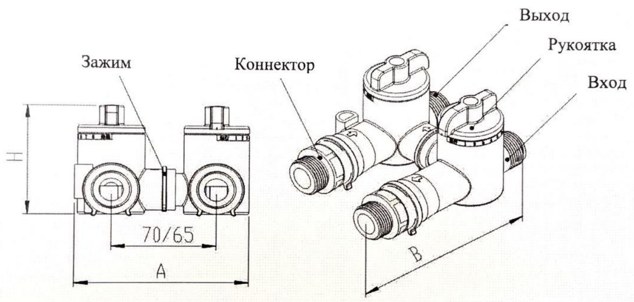
Рис.3 Внешний вид и размеры байпасного клапана TM.F70B.
