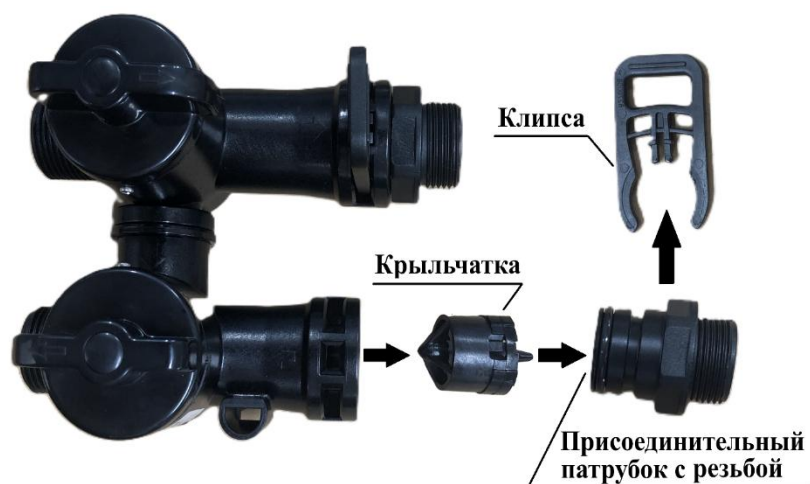
Рис. 5.1 Демонтаж крыльчатки из патрубка очищенной воды байпасного клапана:
