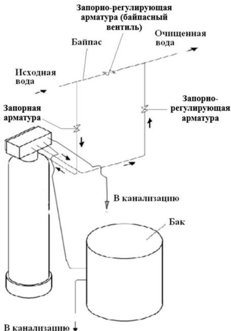
Рисунок 4 — Схема монтажа установки умягчения воды периодического действия WS - 3/4" с обводной линией (байпасом)
