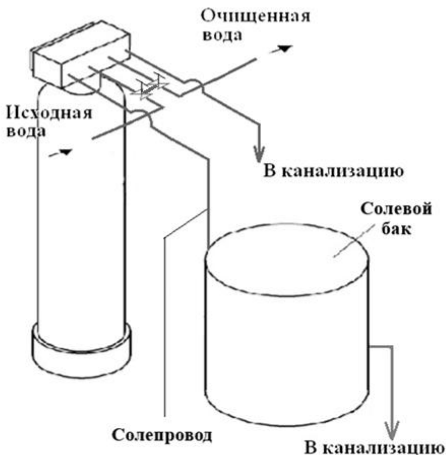
Рисунок 2 — Схема монтажа установки умягчения воды периодического действия WS - 3/4" с байпасным клапаном
