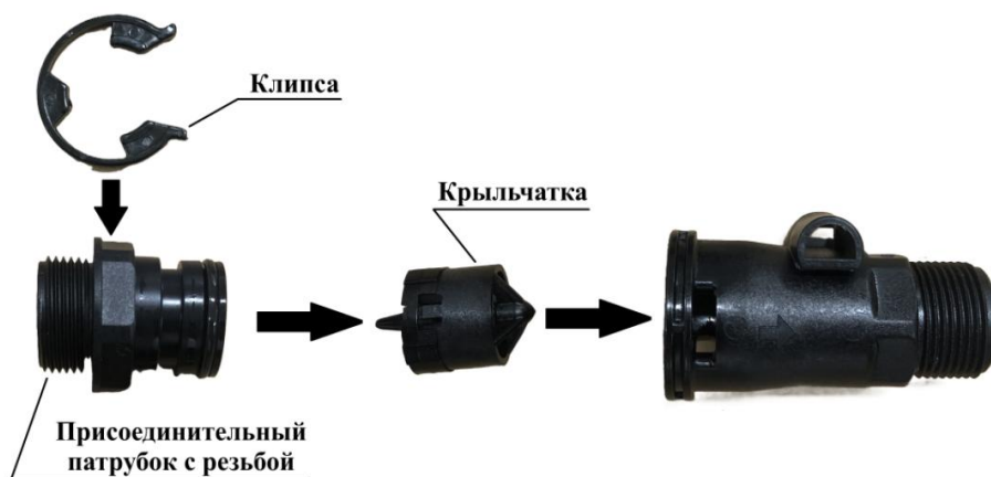
Рис. 5.4 Сборка присоединительного патрубка очищенной воды управляющего клапана с крыльчаткой водосчетчика:
