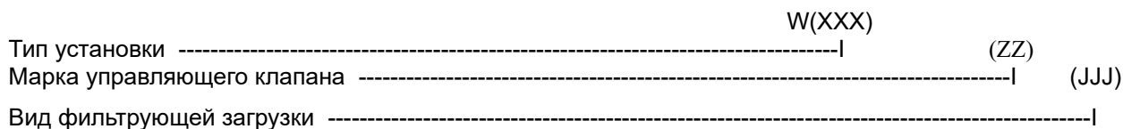
Рисунок 1 — Структура обозначения установки
