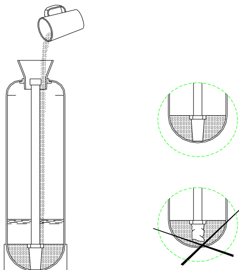
Рис. 4 Порядок загрузки фильтрующего материала в корпус фильтра
