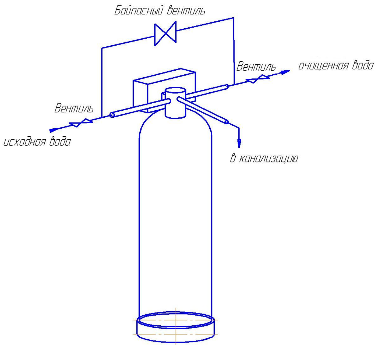
Рисунок 2 — Схема монтажа установки обезжелезивания WFDF с управляющим клапаном Runxin.
