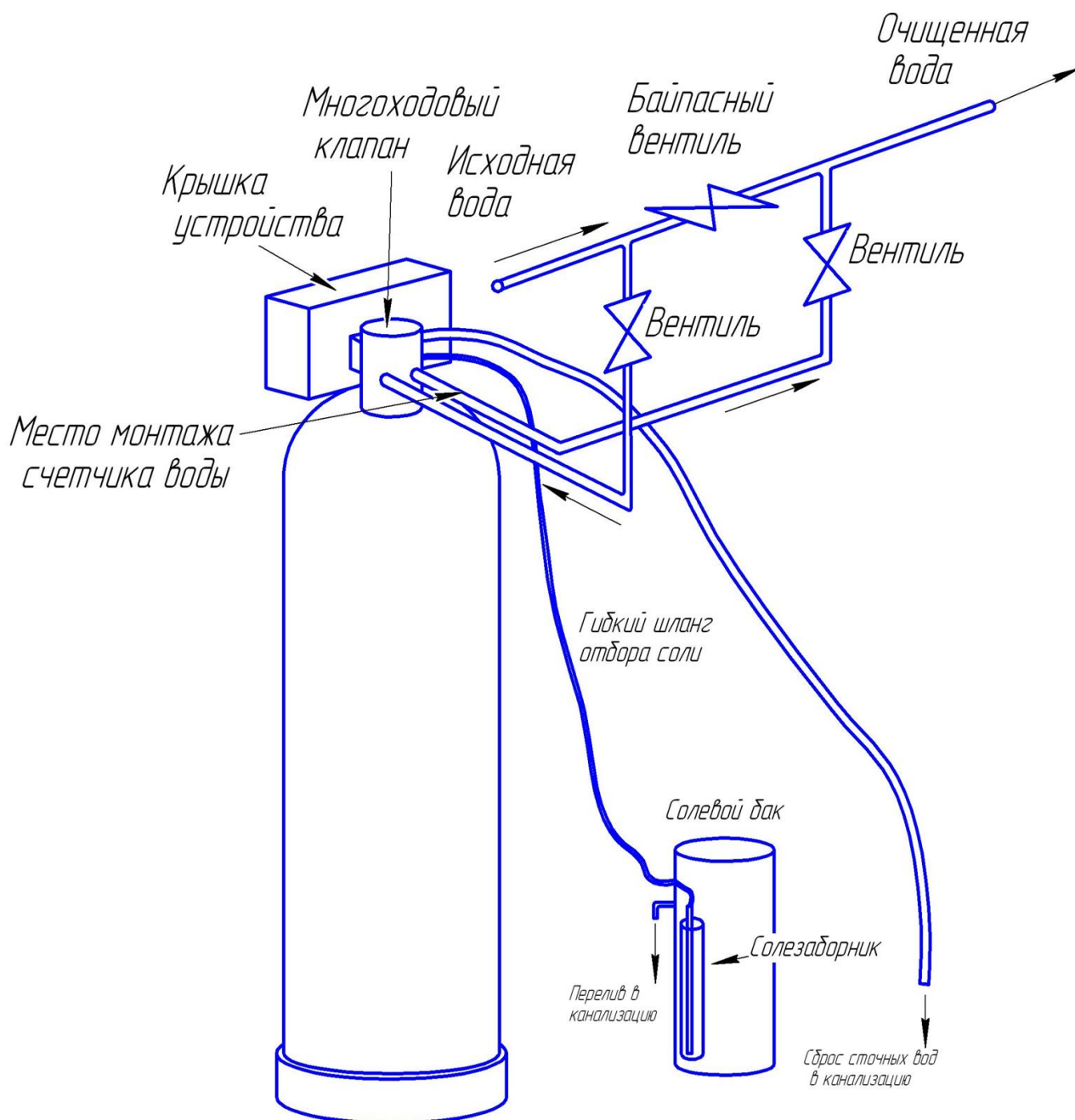
Рисунок 2 — Схема монтажа установки умягчения и обезжелезивания WSDF-0,8...16,5-Rx-(MIX P) подключением \frac{3}{4} ", 1" и 2".
