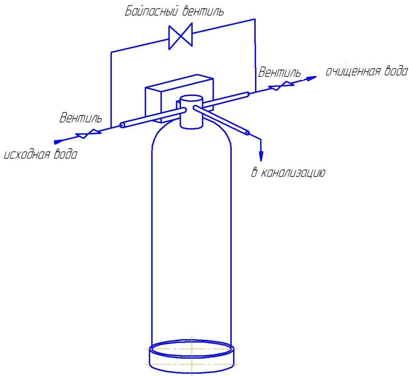
Рисунок 2 — Схема монтажа установки обезжелезивания WFDF с управляющим клапаном Runpin.
