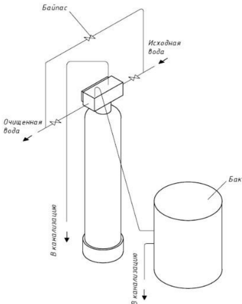
Рисунок 2 – Схема монтажа установки умягчения воды периодического действия WS-5,0-Rx-(BS)...WS-20,0-Rx-(BS)
