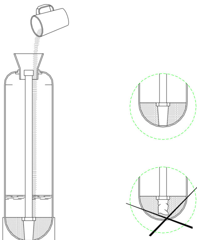
Рисунок 3 — Порядок загрузки фильтрующего материала в корпус фильтра
