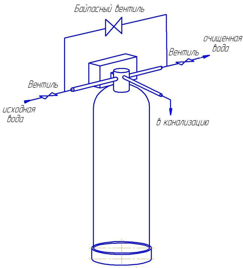
Рисунок 2 — Схема монтажа установки обезжелезивания WFDF-0,5...9,9-RX-(ASIF) подключением 3/4", 1" и 2".
