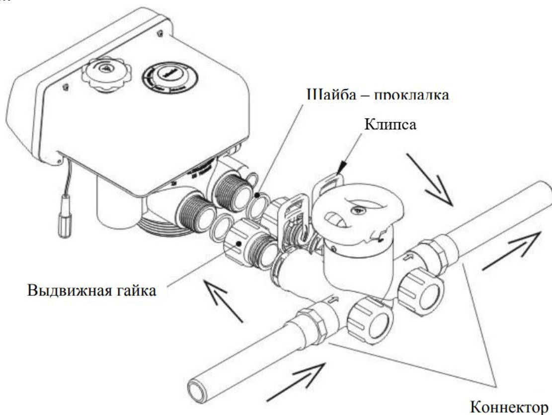
Рис. 3 Установка байпаса-клапана.
