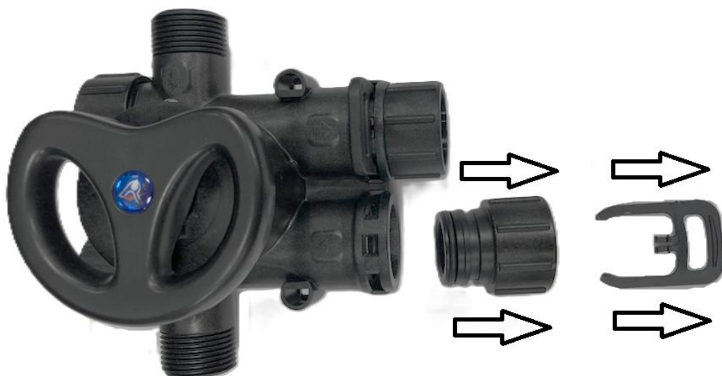
Рис. 6.3 Разборка клапана-байпаса ТМ. F70А с крыльчаткой в сборе: этап 2. Демонтаж присоединительного резьбового фитинга.
