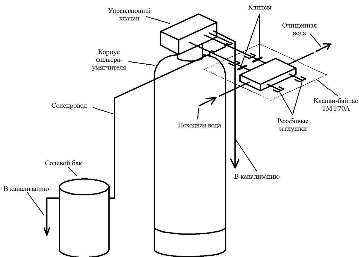
Рис. 4 — Схема монтажа установки умягчения воды периодического действия WS с клапаном байпасом TM.F70A
