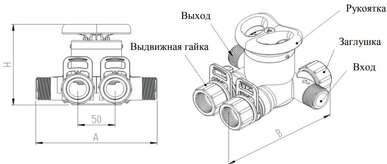
Рис. 2 Внешний вид клапана F70A и его размеры
