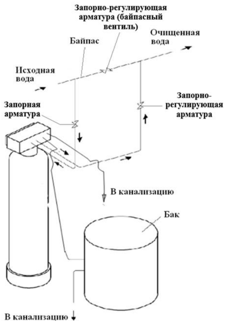
Рисунок 5 — Схема монтажа установки умягчения воды периодического действия WS - 1" с обводной линией (байпасом)
