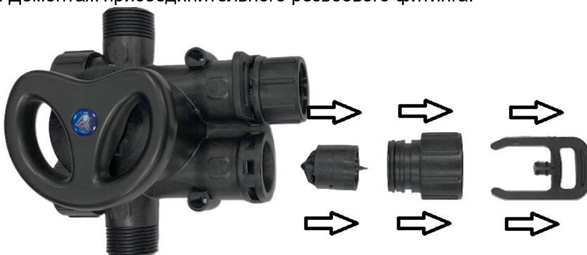
Рис. 6.4 Разборка клапана-байпаса ТМ. F70А с крыльчаткой в сборе: этап 3. Демонтаж крыльчатки водосчетчика.
